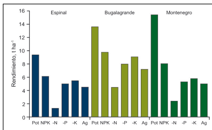
Figura 3. Rendimiento potencial, rendimiento alcanzable, rendimiento de las parcelas de omisión N, P, K y rendimiento del agricultor en tres sitios con diferente condición climática en Colombia.
