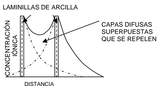
Figura 3. Dispersión del suelo por efecto del traslape de capas difusas.
