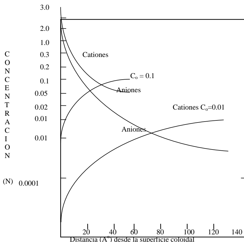
Figura 2. Distribución de cationes y aniones monovalentes cerca a la superficie de una partícula de montmorillonita en función de la concentración. (Adaptado por Bohn et al, 1979 de Nielson et al. , 1972.).
