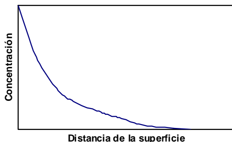
Figura 1. La Doble Capa Difusa.
